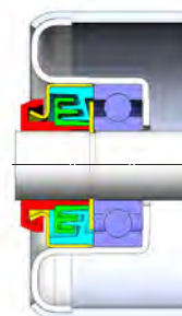
C : Sertissage boîtier à aile retournée
