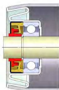
B : Sertissage boîtier tôle en S
