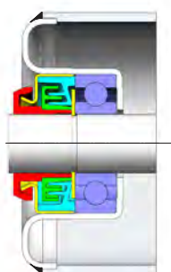
D : Soudure boîtier tôle à aile retournée
