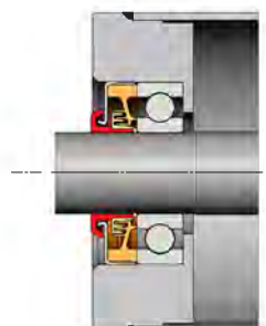
H : Soudure boîtier massif en pleine jupe
