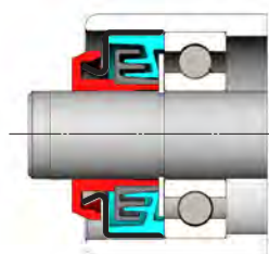
A : Liaison sans boîtier
