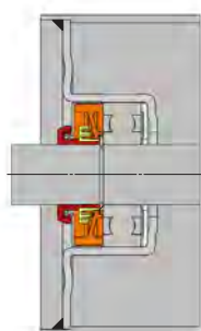
F : Soudure boîtier à aile plate à l'intérieur du tube
