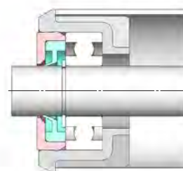
I : Emmanchement boîtier plastique
