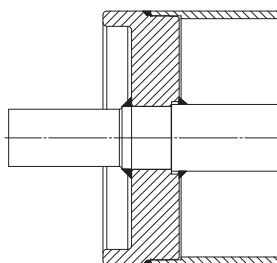
Tambour à arbre soudé
