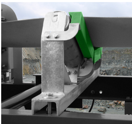
Support pour rouleaux équipé d'Optim'Protec-RS
