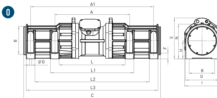
SPÉCIFICATIONS DIMENSIONNELLES (mm)
