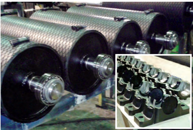
Plaatsing van lagers direct op de assen
