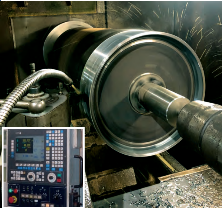
Bewerking van de trommelstructuur met onze numerieke machines
